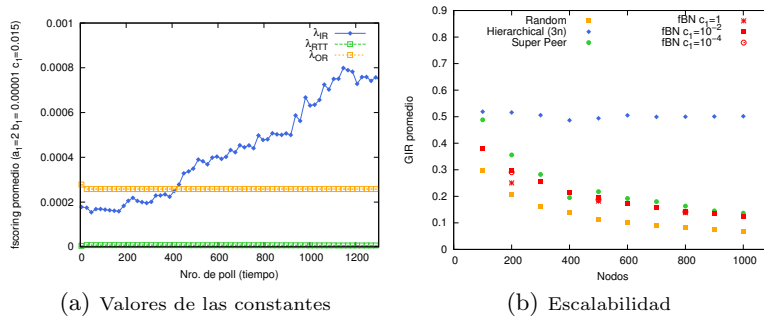
Figura 5: \lambda_{\text{OR}} es constante, con valores varios órdenes de magnitud mayor que \lambda_{\text{IR}} . Como en el caso anterior se agrega una constante a \lambda_{\text{OR}} (denominada c_1 ) para equiparar los valores desde el inicio de la simulación. Se calculan para cada una de las magnitudes que intervienen en la función de scoring el promedio de todos los vecinos para los que se calcula la función en un nodo determinado y se observa su evolución en el tiempo. La Figura (a) muestra los promedios una vez agregada la constante. (b) GIR promedio para las políticas de distribución Jerárquica, Super Peer (5-SP), Random y fBN: a_1 = 1, b_1 = 10^{-4}, c_1 = 1, 10^{-2}, 10^{-4} , para redes de topología Exponencial con distintas cantidades de nodos (100 a 1000 nodos).
