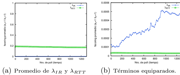
Figura 12: Al normalizar, \lambda_{IR} sigue siendo una función creciente, pero que crece muy suavemente, mientras que \lambda_{RTT} es casi constante con valores varios órdenes de magnitud mayor. Al tener \lambda_{IR} una pendiente tan suave la mayor parte del tiempo quedan invertidas las prioridades, teniendo más peso RTT que la información de recursos, aunque al ser está última creciente y acotada entre 0 y 1, en algún momento comenzará a tomar valores mayores o iguales que RTT. Una forma de forzar esta condición es agregar una constante al segundo término, \lambda_{RTT} , que permita equiparar los valores desde el inicio de la simulación. En las Figuras (a) se pueden observar los resultados de cada una de las magnitudes que intervienen en la función de scoring en función del tiempo, tomando el promedio de todos los vecinos para los que se calcula la función en un nodo determinado. En la Figura (b) se ven los promedios una vez agregada la constante.
