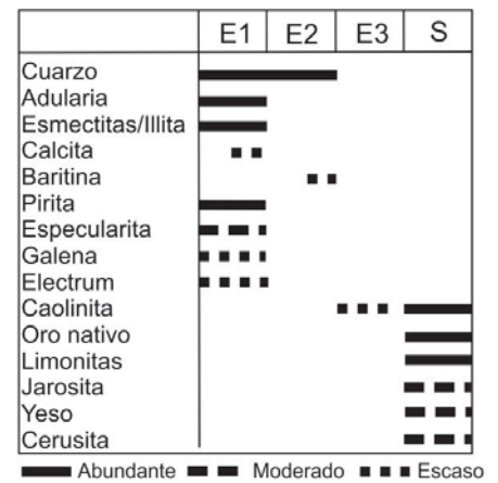
Figura 4: Diagrama paragenético del relleno hidrotermal que conforma el cemento de la brecha. E1: etapa 1, E2: etapa 2, E3: etapa 3; S: alteración supergénica.
