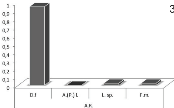
Figs 1-3. The Berger Parker dominance index: 1, in size 1; 2, in size 2; 3, in size 3 [A. (P.) l., Ascocotyle (Phagicola) longa ; D. f., Dicrogaster fastigata ; E. a., Ergasilus atafonensis ; E. v., Ergasilus versicolor ; F. m., Floridosentis mugilis ; H. m., Hymenocotta manteri ; L. sp., Ligophorus sp.; M. m., Macrocotyle macracantha ; H. gen. sp., Metacercariae Hemiuridae gen. sp.; M. p., Microcotyle pseudomugilis ; M. u., Myzobdella uruguayensis ; P. sp. 1, Parabrachiella sp. 1; P. sp. 2, Parabrachiella sp. 2; P. m., Phyllodistomum mugilis ].
